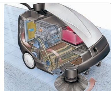
Esquema funcionamiento mod. 710 a baterías.
